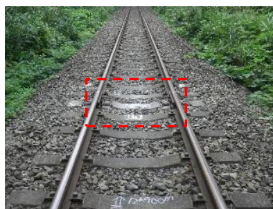
劣化による沈下
