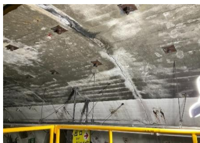
トンネル内頂部の補修・修繕箇所調査（葛老山トンネル他）
