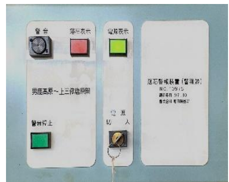
落石検知表示装置
