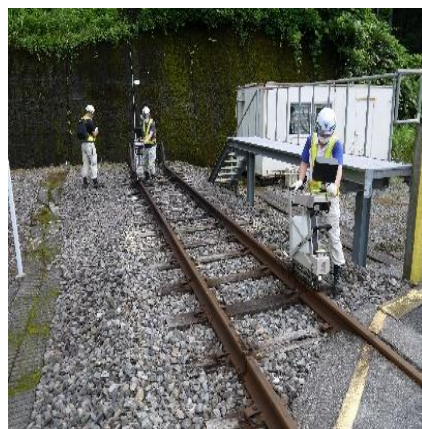
手押し式の超音波探傷検査
